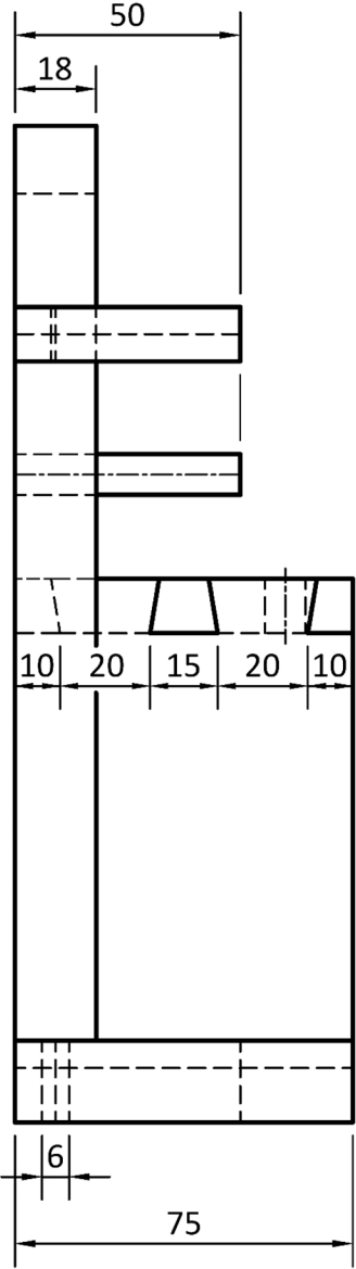
End View/Taobhchló
